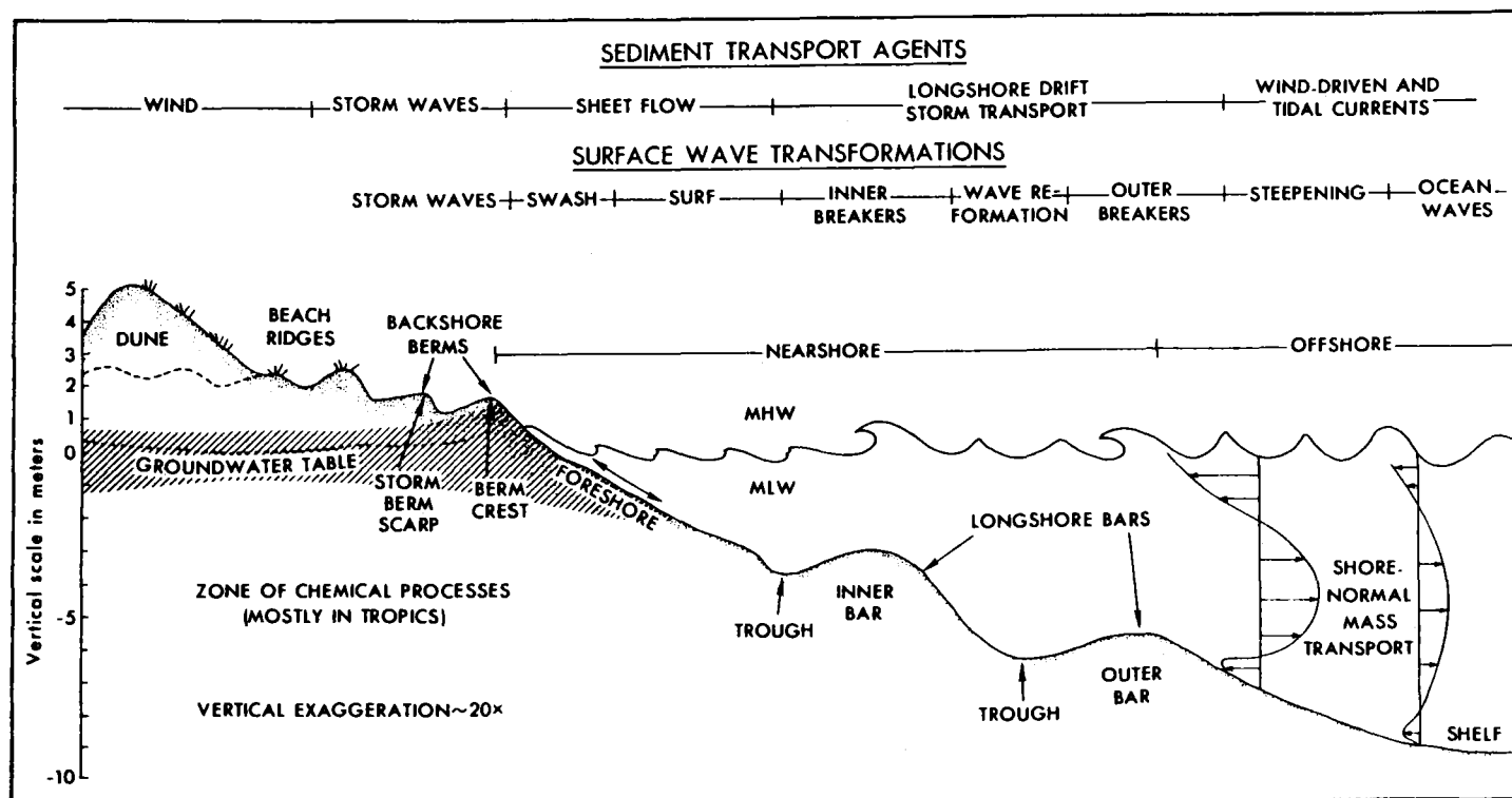
Figure 32: Profil de côte sablonneuse définissant des composants géomorphologiques et des procédés physiques
