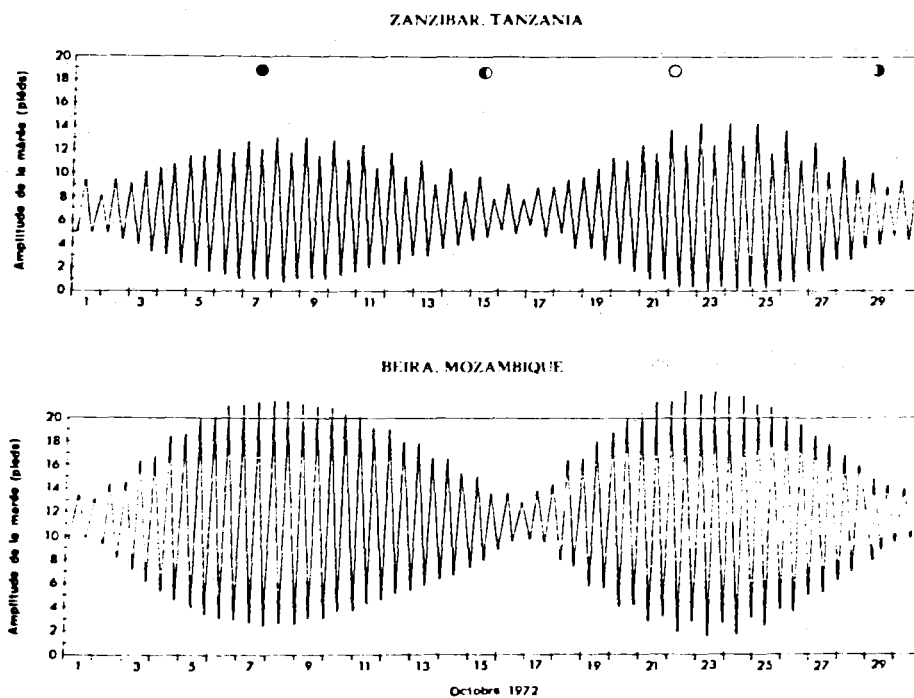
Figure 28: Amplitudes des marées au cours d'un cycle mensuel: • : nouvelle
