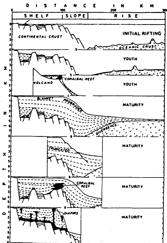
Figure 19: Etapes du développement évolutif des marges continentales. Exagération verticale \pm 10\times (d'après Emery, 1980)
