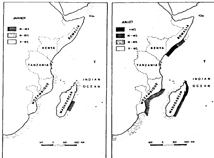
Figure 22: Fréquence des vents de mer à vélocité plus grande que 12 miles/heure (d'après Orme, 1982)
