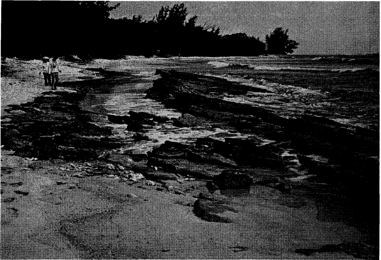
Figure 35: Dépôts de plage indurés dans la zone de marnage sur une plage sablonneuse. A noter les unités d'acréction originales de la plage, maintenant préservées par le processus de lithification. Ce processus s'effectue très rapidement (au cours de quelques dizaines d'années)
