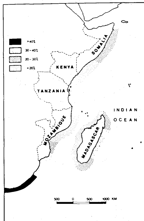
Figure 30: Principales forces génératrices des vagues (d'après Hayden et autres, 1973)
