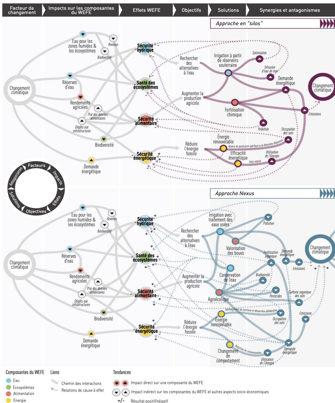
Figure RID2 | Impacts, interactions et effets en cascade des facteurs de changement et des solutions sur les éléments eau, énergie, alimentation et écosystèmes. Le changement climatique a un impact sur les composantes du nexus eau-énergie-alimentation-écosystèmes. Pour garantir la sécurité hydrique, énergétique, et alimentaire ainsi que la santé des écosystèmes, les décideurs politiques doivent trouver des solutions adaptées. Les solutions développées selon une approche cloisonnée pourraient renforcer les antagonismes, avoir un impact négatif sur l'eau, l'énergie, l'alimentation et les écosystèmes et accroître le changement climatique. Une approche nexus, en intégrant la complexité des interactions, peut réduire considérablement les antagonismes, maximiser les synergies et promouvoir des résultats positifs sur les composantes du nexus.
