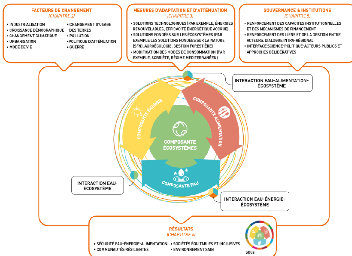
Figure RID1 | Schéma du principe du nexus eau-énergie-alimentation-écosystèmes et des résultats du rapport pour le bassin méditerranéen. Divers facteurs de changement, directs et indirects, impactent les composantes eau-énergie-alimentation-écosystèmes. Le WEF E comporte une série d'interactions à deux, trois niveaux et plus, qui doivent être abordées par une gouvernance et des institutions appropriées, capables de développer des actions d'adaptation et d'atténuation qui favorisent les synergies pour atteindre la sécurité de l'eau, de l'alimentation, de l'énergie et la santé des écosystèmes conformément aux ODD.
