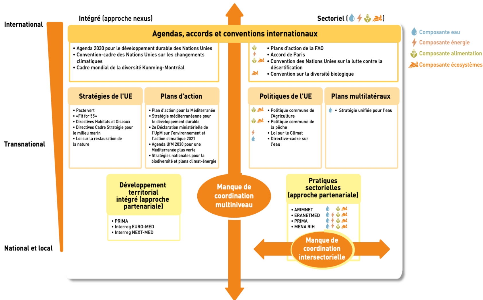
Figure RID5 | Politiques intégrées et sectorielles à plusieurs niveaux sur le nexus eau-énergie-alimentation-écosystèmes en Méditerranée (voir {5.3.1 ; 5.3.3} pour la description des programmes AIMNET, ERANETMED, MENA RIH et PRIMA).
