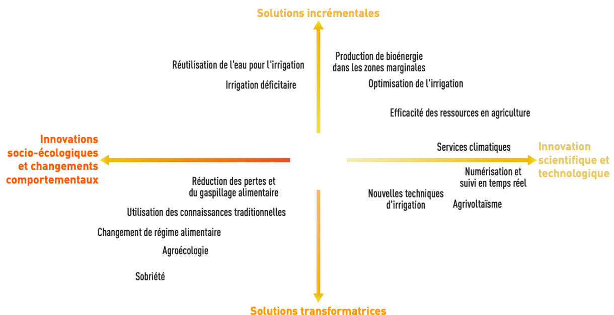
Figure RID3 | Quadrant des solutions intégrées d'adaptation et d'atténuation de type nexus pour l'eau, l'énergie, l'alimentation et les écosystèmes, mises en œuvre dans la région méditerranéenne. Les solutions d'adaptation et d'atténuation vont des solutions incrémentales aux solutions transformatrices, et de l'innovation scientifique et technologique aux innovations socio-écologiques et au changement de comportement.
