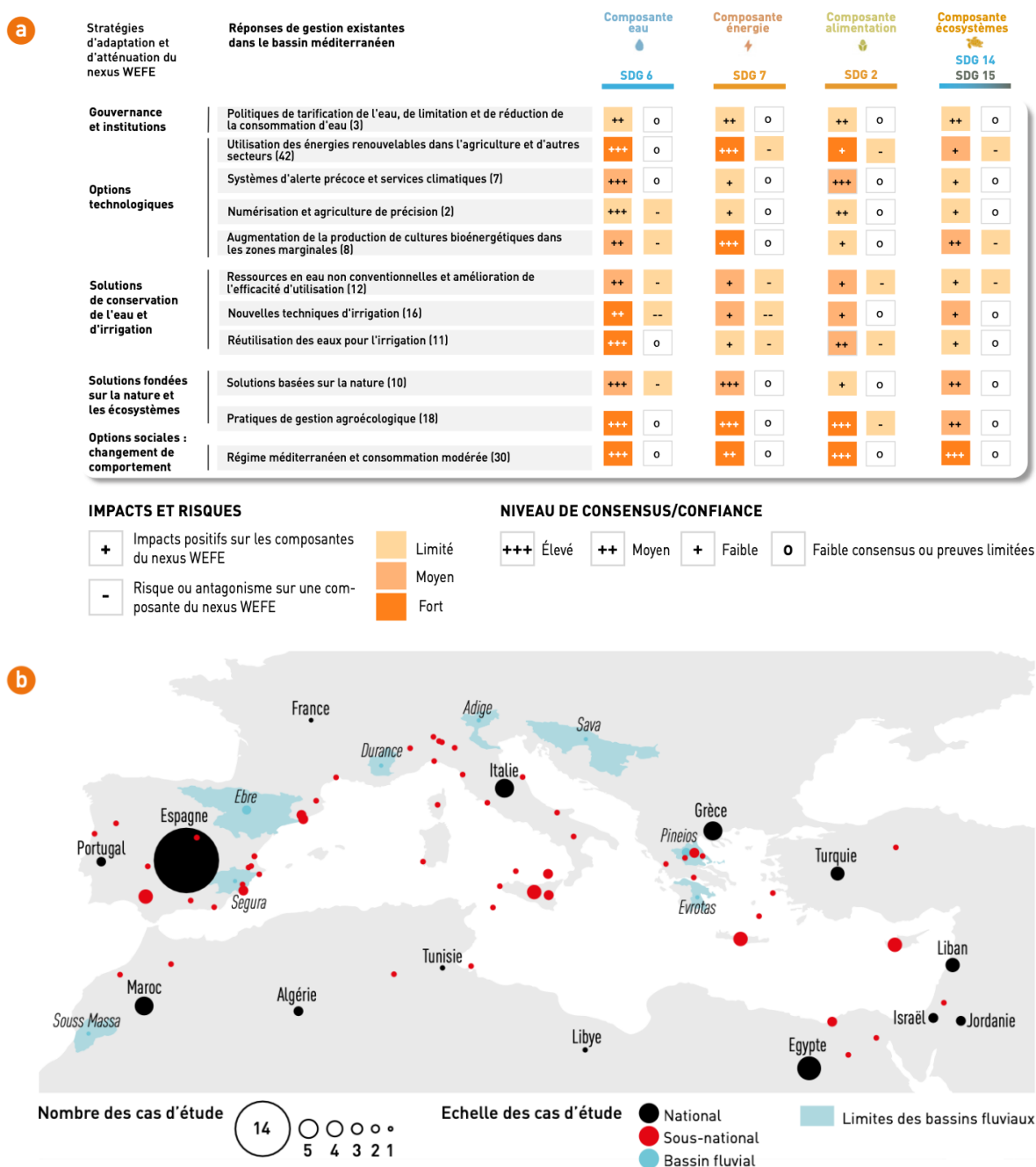
Figure RID4 | (a) Évaluation des principaux impacts et antagonismes des solutions intégrées d'adaptation et d'atténuation de type nexus pour l'eau, l'énergie, l'alimentation et les écosystèmes, mises en œuvre dans les pays méditerranéens. Le lien est établi avec les ODD par le biais des composantes du nexus. Les chiffres entre parenthèses correspondent au nombre d'articles étudiés pour évaluer chaque solution. Le niveau de preuves est quantifié par le nombre d'articles examinés (indiqués par des chiffres entre parenthèses et classés en trois catégories : limitées en orange pâle, moyennes en orange et solides en orange foncé), tandis que le degré de consensus mesure l'accord entre les articles (o pour un faible consensus ou des preuves limitées, + pour un faible niveau de consensus/preuves, ++ pour un niveau moyen et +++ pour un niveau élevé). Ce tableau ne passe pas en revue toutes les solutions possibles, mais celles qui ont été mises en œuvre en Méditerranée, rapportées dans la littérature scientifique et évaluées dans le rapport. (b) Répartition spatiale des études de cas examinées.
