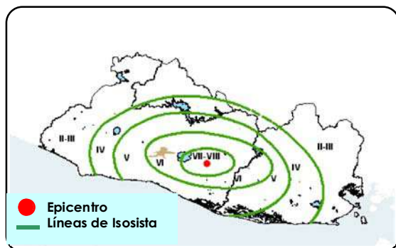
Mapa 2-7: Isosistas del terremoto del 13S de Febrero de 2001
