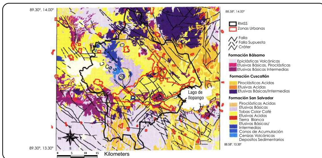
Mapa 2-8: Geología de la RMSS
