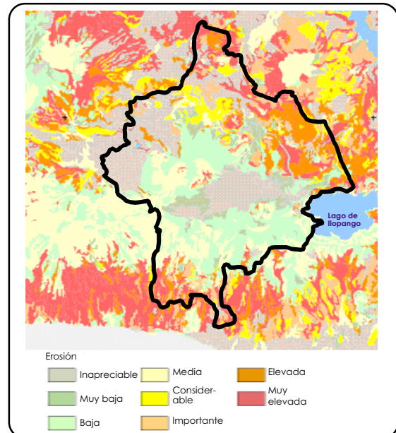
Mapa 2-39: Erosión de los suelos en la RMSS
