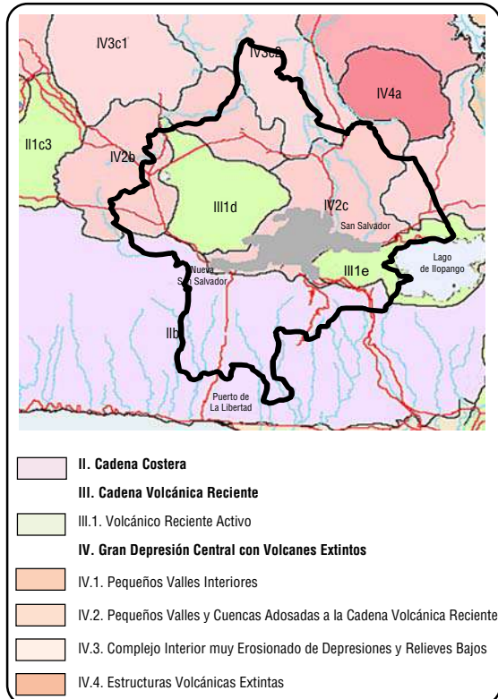
Mapa 2-4: Unidades morfoestructurales en la RMSS
