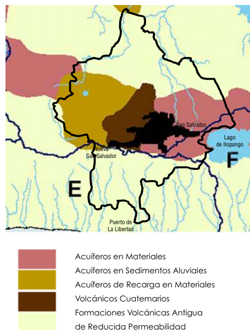
Mapa 2-25: Mapa Hidrogeológico, RMSSS
