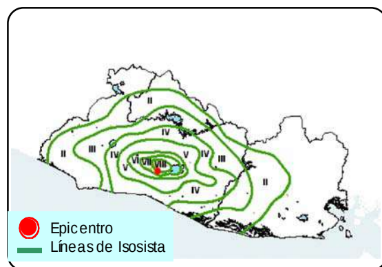
Mapa 2-5: Isosistas del terremoto del 10 de Octubre de 1986
