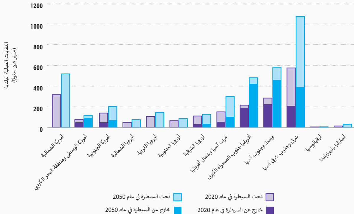
الشكل 2: توليد النفايات الصلبة البلدية ومقدار ما هو خارج عن السيطرة من هذه النفايات في عام 2020، مع توقعات لعام 2050 ما لم تُتخذ إجراءات عاجلة
