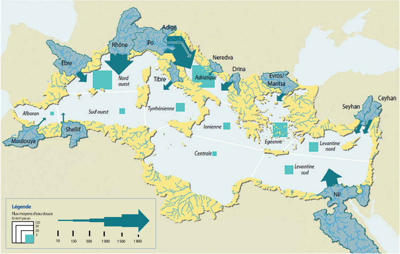
DÉVERSEMENT D'EAUX DOUCES D'ORIGINE FLUVIALE EN MÉDITERRANÉE
