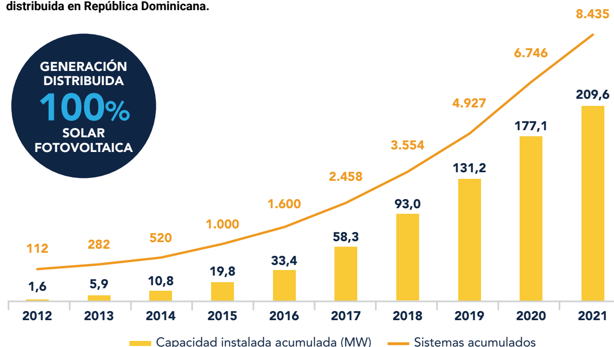
Gráfico 46. Evolución de la capacidad instalada (MW) y cantidad de sistemas de generación distribuida en República Dominicana.
