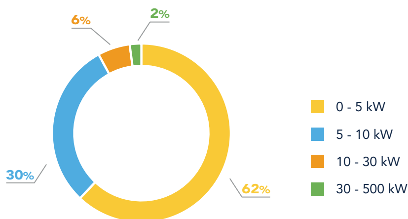
Gráfico 36. Distribución de la capacidad instalada en función al tamaño del sistema - México.
