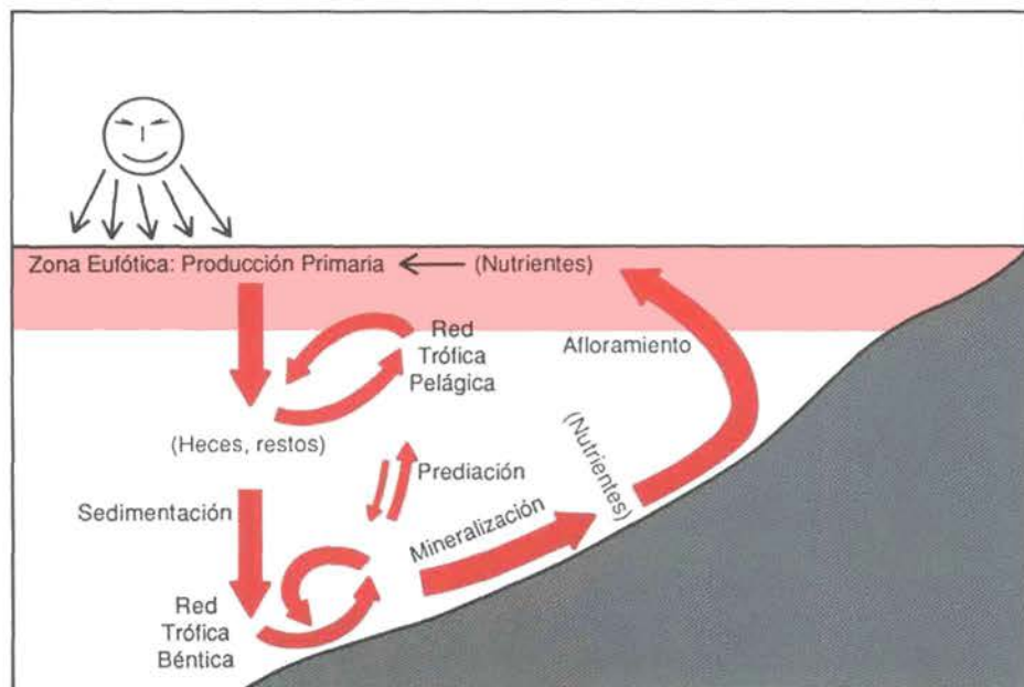
Fig. 1.5 Esquema de afloramiento, mostrando la estrecha conexión entre los subsistemas bentico y pelágico. (Schematic of upwelling showing the tight connection between the benthic and pelagic subsystems.) (Adapted from El Niño: Su Impacto en la Fauna Marina, IMPARE, Peru, 1985 )
