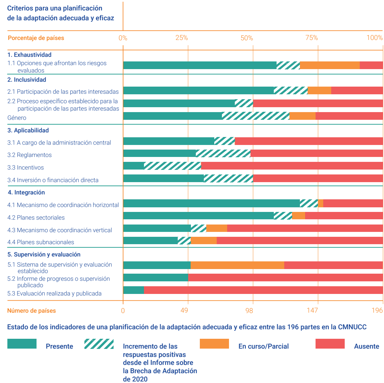
Figura ES.2 Evaluación de la adecuación y eficacia de la planificación de la adaptación a escala mundial
