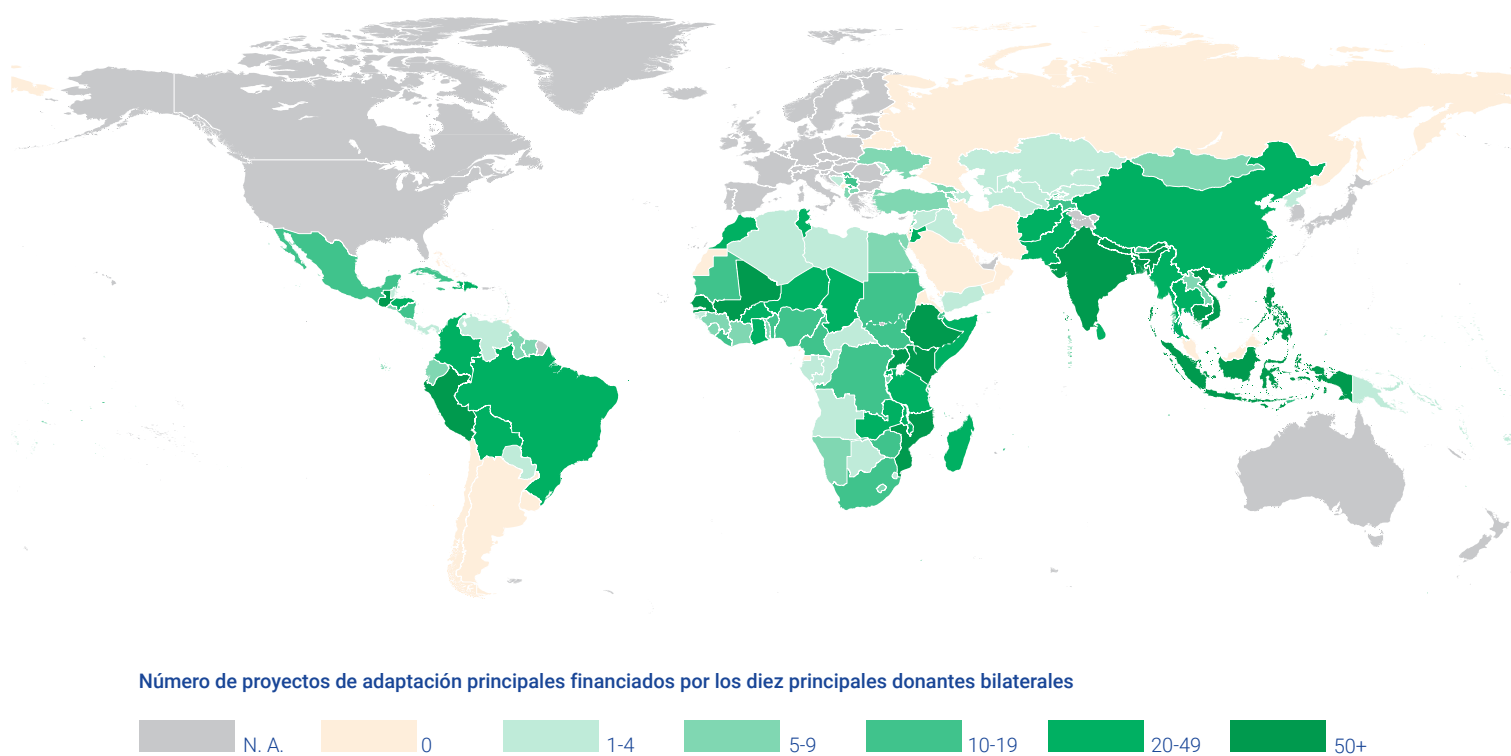
Figura ES.5 Distribución geográfica de los proyectos de adaptación principales financiados por los diez principales donantes bilaterales
