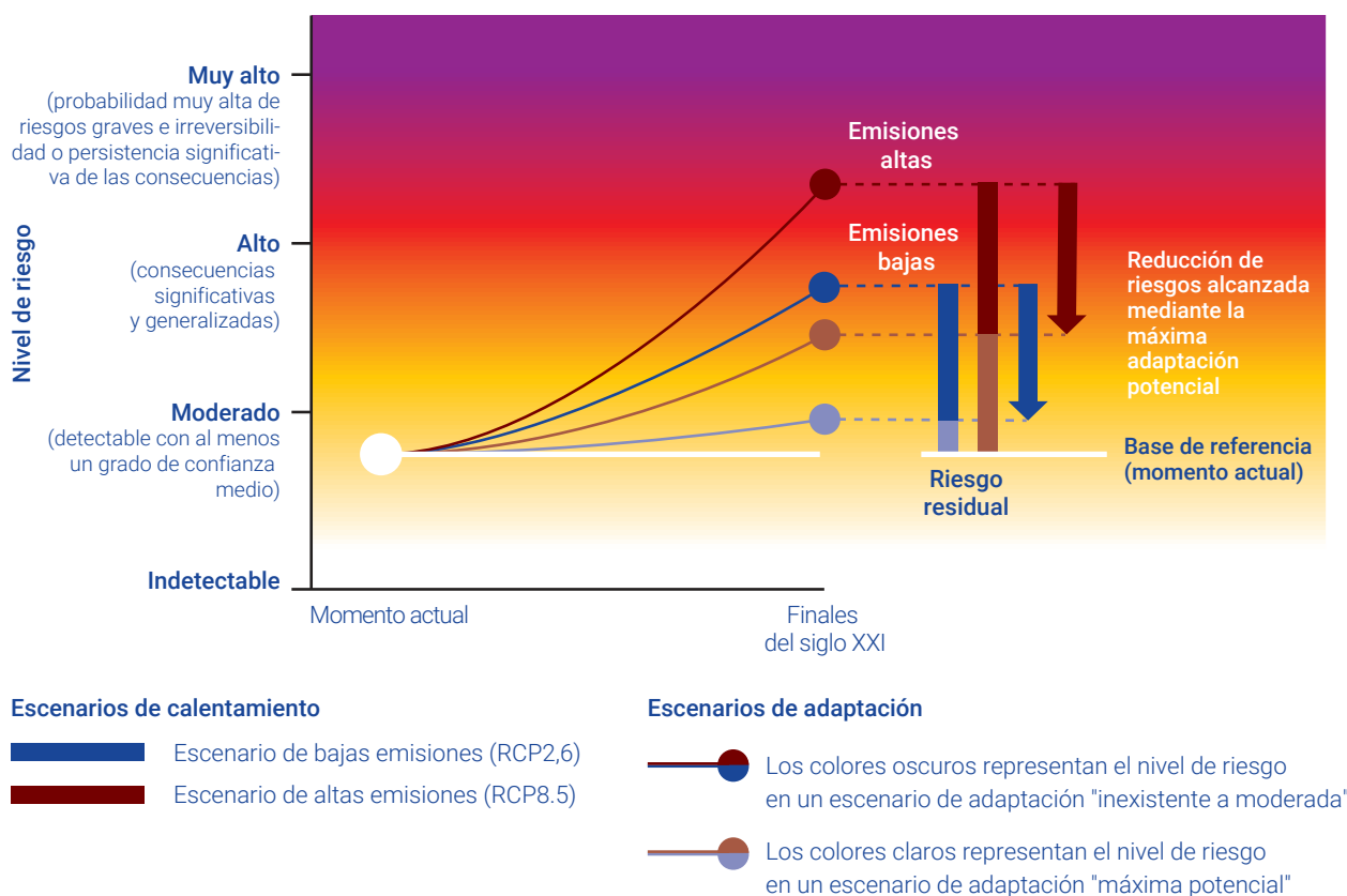
Figura ES.7 Resultados de la adaptación según la información publicada en los informes especiales correspondientes al ciclo del sexto informe de evaluación del IPCC sobre la criosfera en tierra y en los océanos
