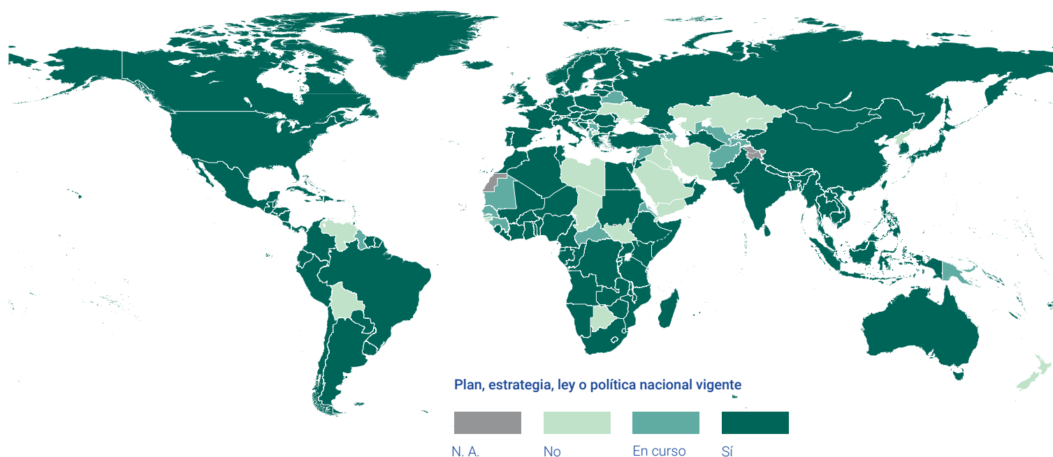
Figura ES.1 Estado de la planificación de la adaptación a escala mundial, a 5 de agosto de 2021
