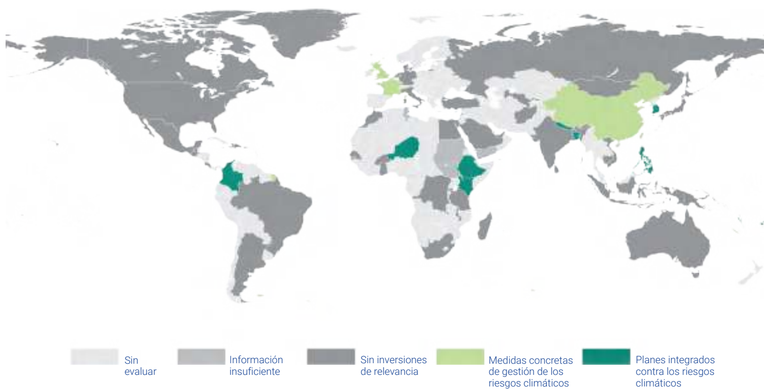
Figura ES.6 Países con intervenciones de adaptación concretas en los paquetes de estímulo, a 31 de enero de 2021
