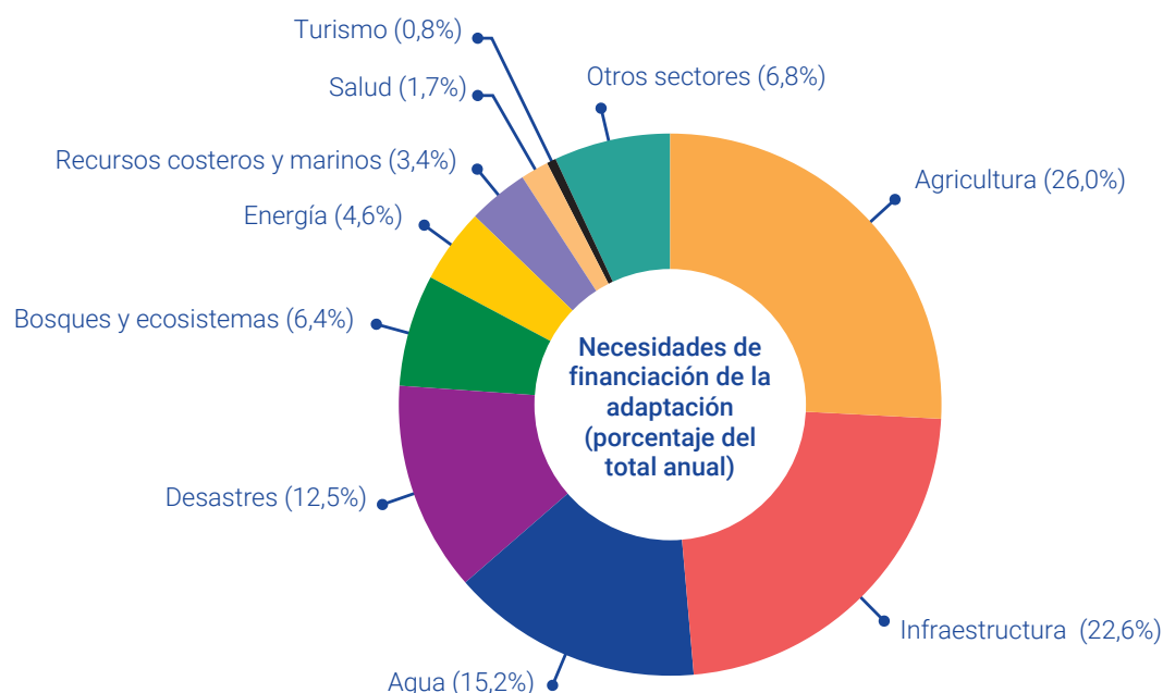
Figura ES.3 Necesidades de financiación de la adaptación por sectores, en función de las contribuciones determinadas a nivel nacional y los planes nacionales de adaptación de 26 países en desarrollo
