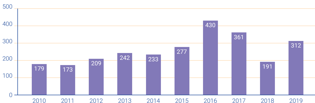
Figura ES.4 Número de proyectos de adaptación principales nuevos iniciados al año con financiación de los diez principales donantes para la adaptación
