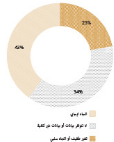
الشكل هـ- اتجاه بيانات مؤشرات أهداف التنمية المستدامة المتصلة بالبيئة، على الصعيد العالمي
