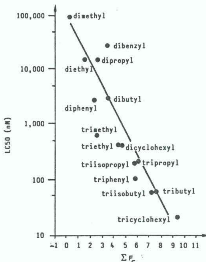
Fig. 15 Corrélation entre les valeurs de la CL_{50} de larves du crabe Rhithropanopeus harrisii (durée d'exposition: 10-12 jours) et la constante de Leo (un indice du comportement hydrophobe) pour certains homologues di- et triorganostanniques. D'après Laughlin et Linden (1985)
