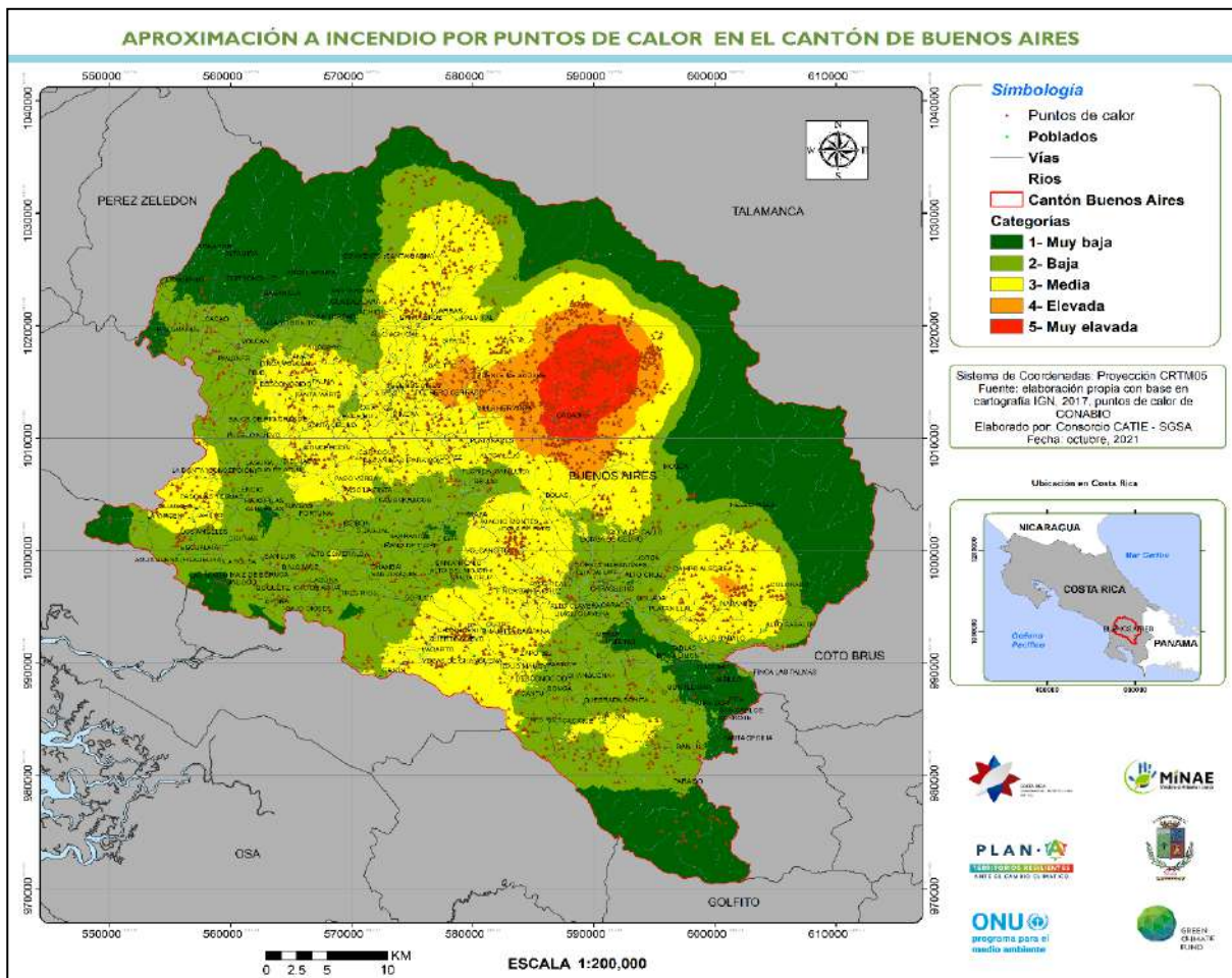
Figura 23. Incendios forestales en el cantón de Buenos Aires
