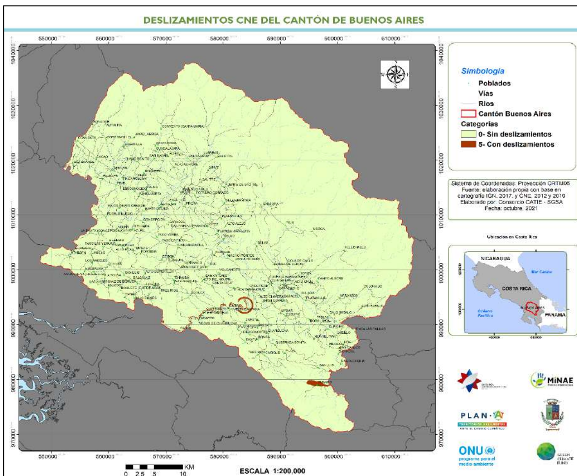
Figura 18. Inestabilidad de laderas en el cantón de Buenos Aires (Fuente: CNE, en SNIT 11 )
