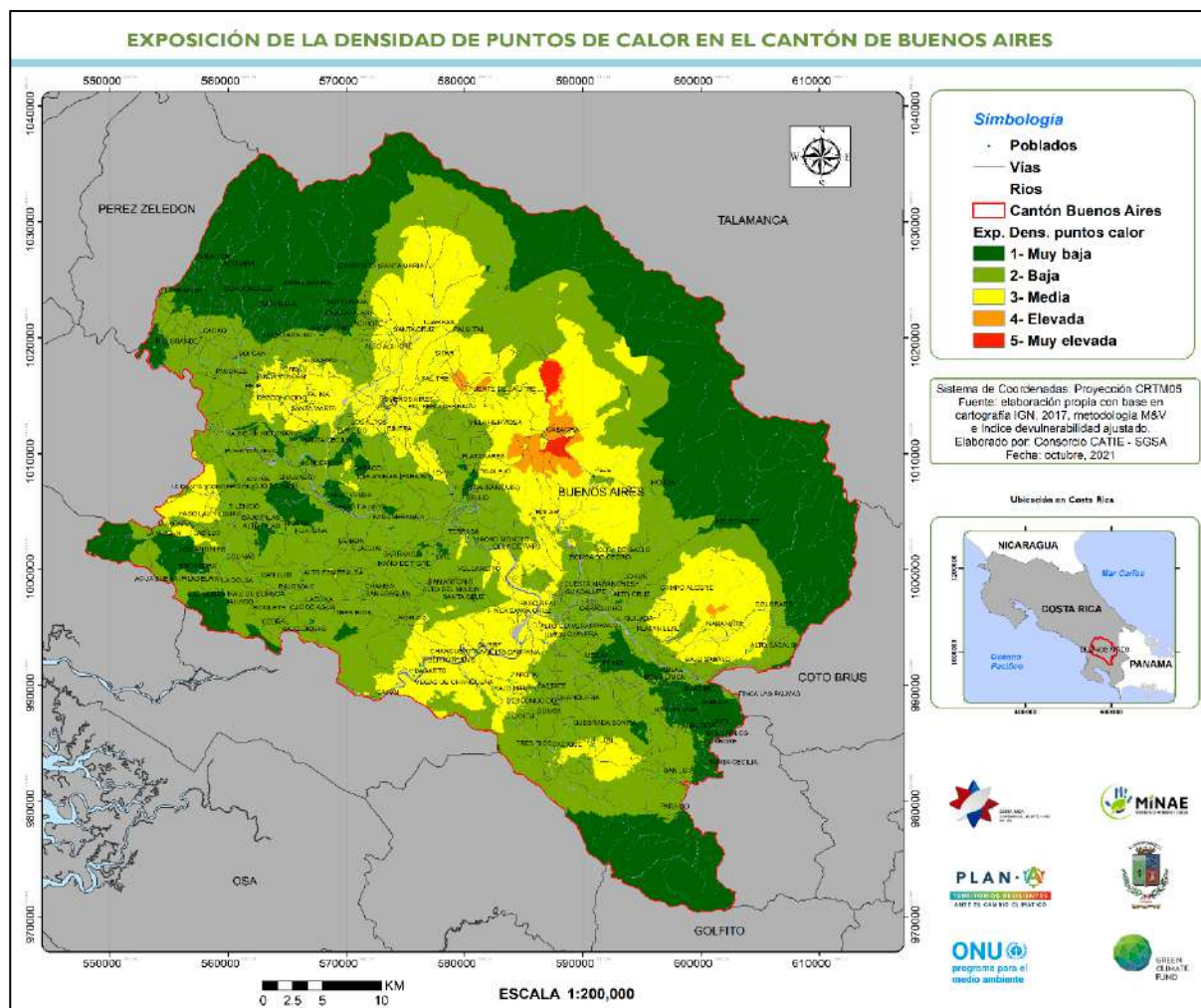
Figura A.5.4. Exposición a la densidad de puntos de calor, en el cantón de Buenos Aires.
