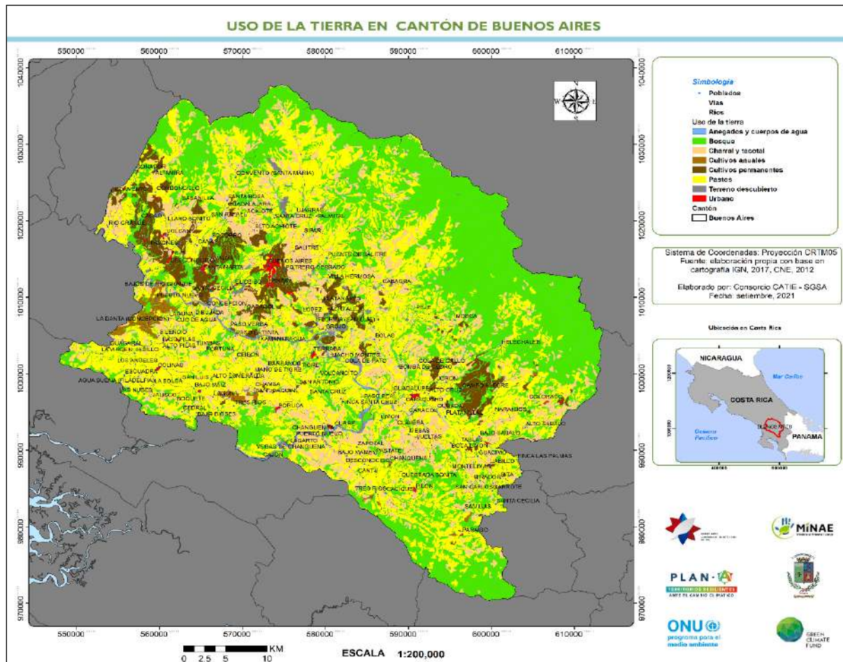
Figura 14. Uso de la tierra en el cantón de Buenos Aires
