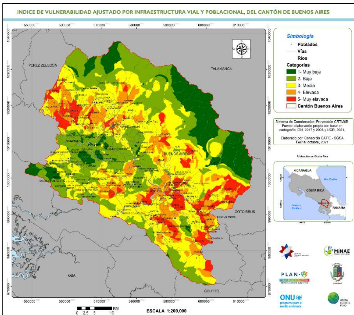
Figura 36. Índice de vulnerabilidad ajustado por infraestructura y vialidad del cantón de Buenos Aires.
