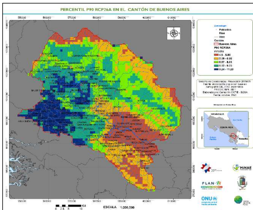
Figura 28. Percentil 90 RCP2.6A, horizonte cercano
