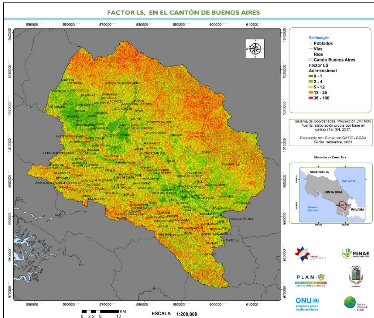
Figura A.3- 5. Factor LS en el cantón de Buenos Aires
