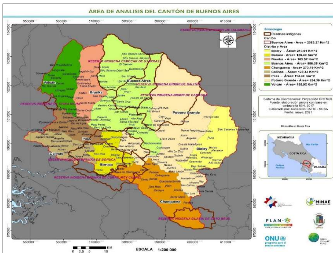
Figura 2. Cantón de Buenos Aires, distritos y reservas indígenas
