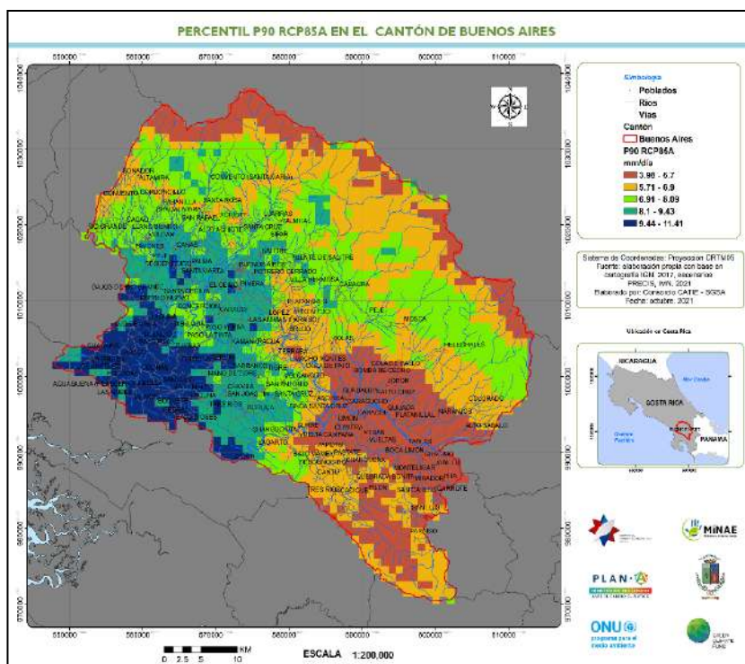
Figura 30. Percentil 90 RCP8.5A, horizonte cercano
