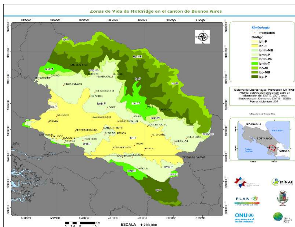
Figura 13. Zonas de vida en el cantón de Buenos Aires Fuente: Elaboración propia, con base información CATIE (CCT, 1990)
