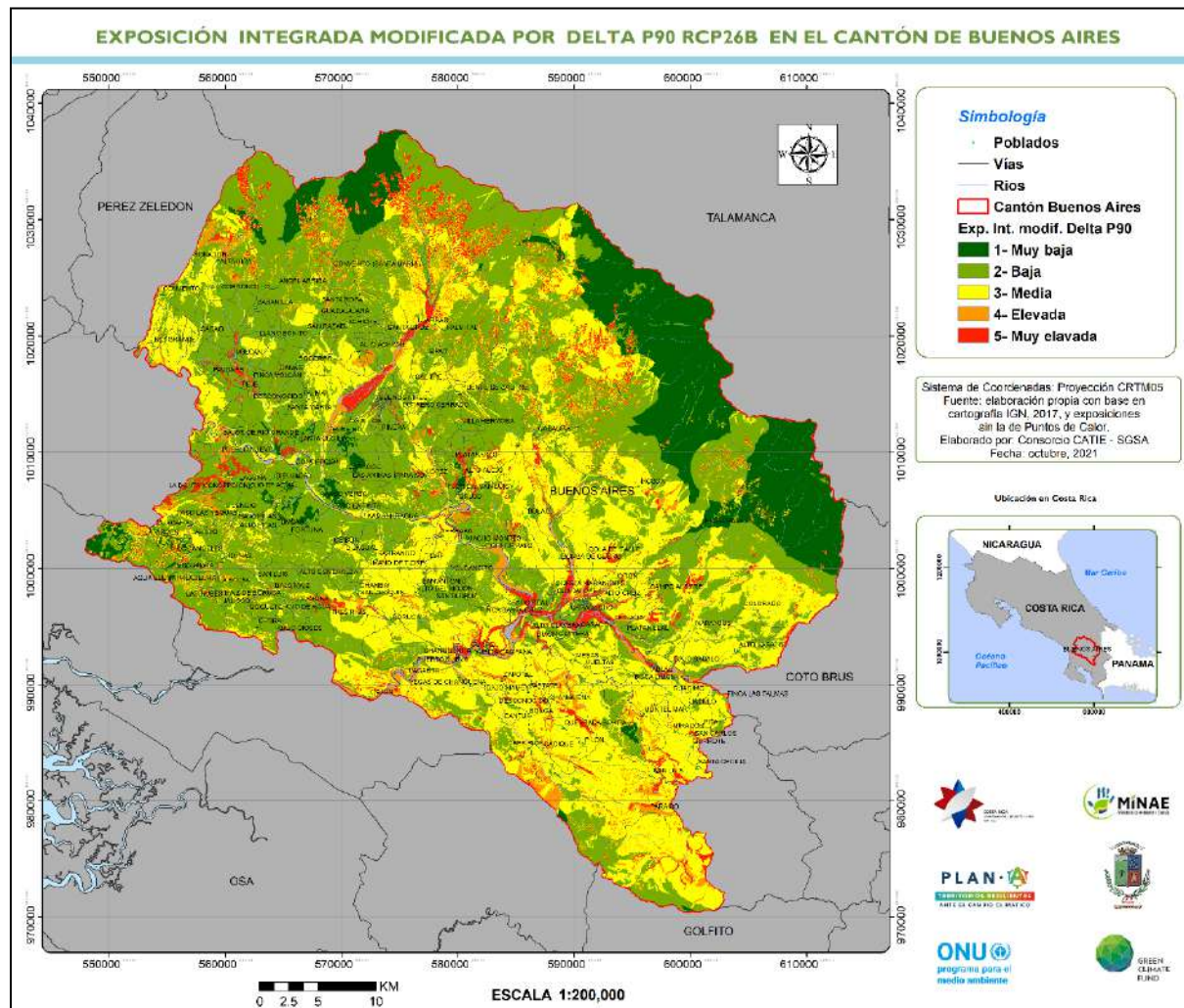
Figura 38. Exposición futura por escenario P90 RCP2.6B en el cantón de Buenos Aires
