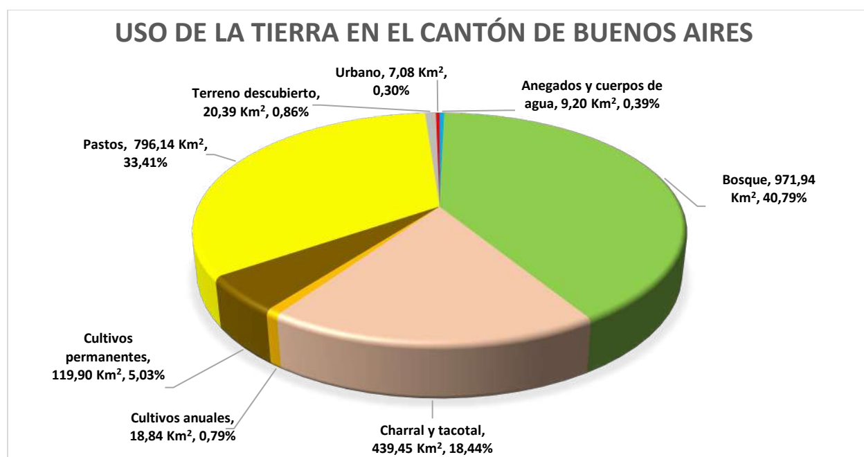
Figura 15. Áreas de los principales usos de la tierra en el cantón de Buenos Aires
