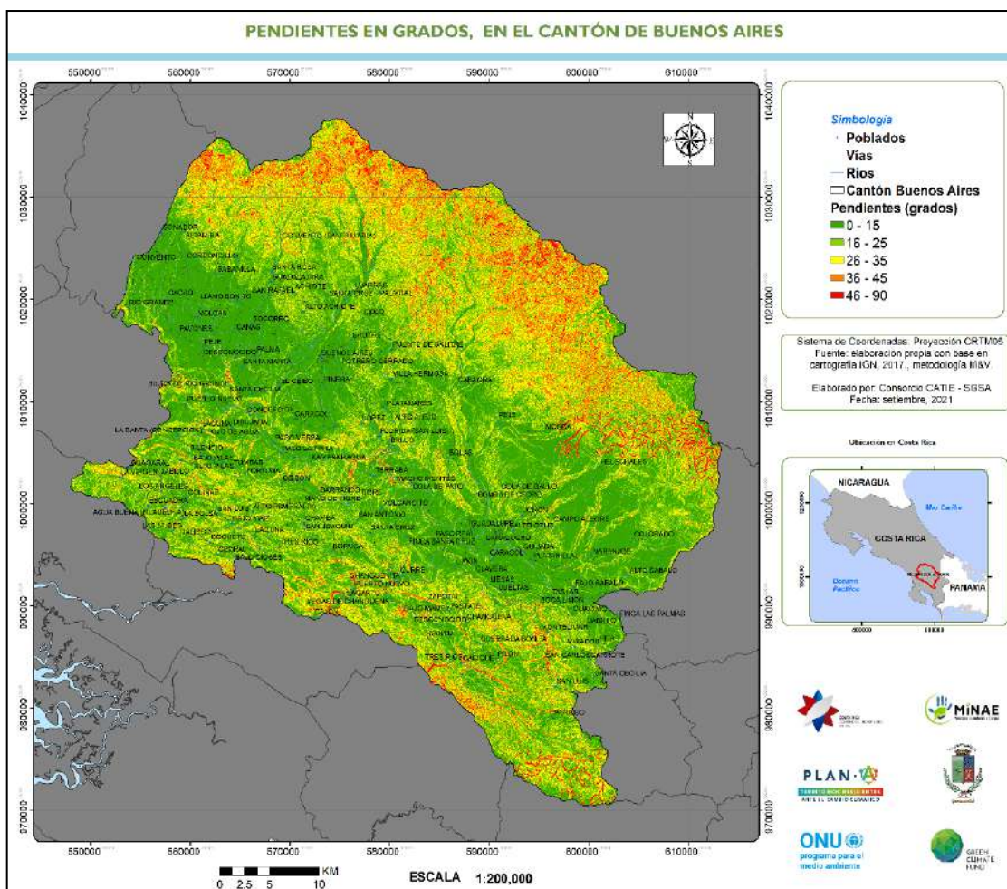
Figura A.2-2. Pendientes, en grados, en el cantón de Buenos Aires
