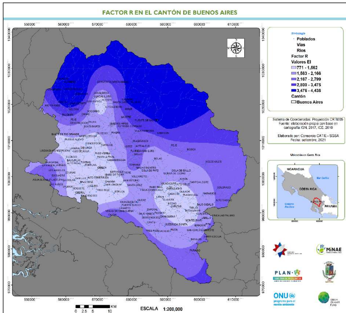
Figura A.3- 1. Factor R (erosividad de la lluvia), cantón de Buenos Aires. Fuente: elaboración propia con modelo de Vahrson, estimado por ICE, 2010.
