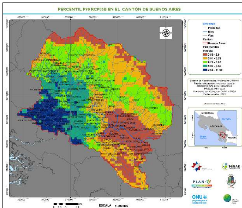
Figura 31. Percentil 90 RCP8.5B, horizonte medio
