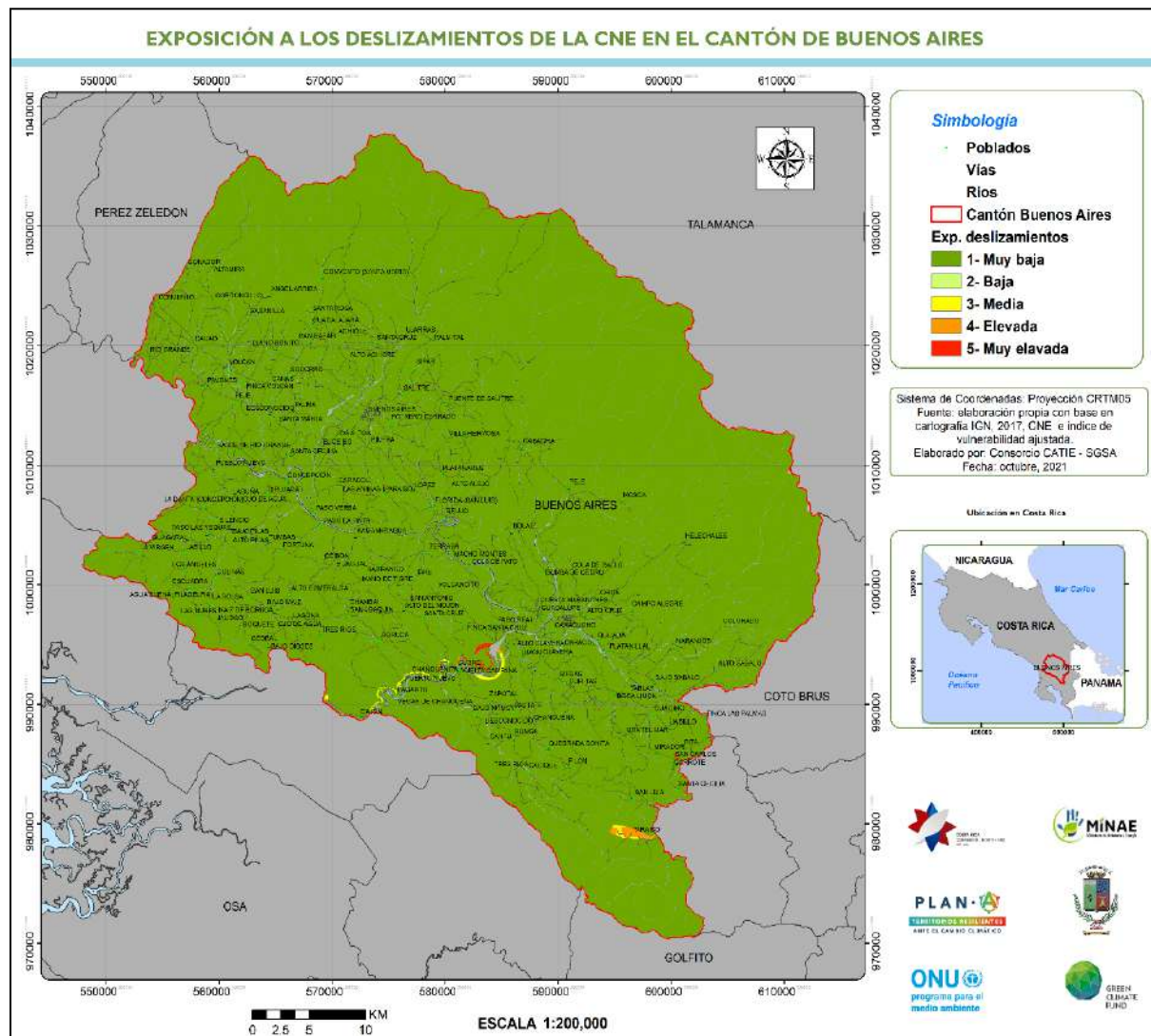
Figura A.5.2. Exposición a la inestabilidad de laderas de la CNE, en el cantón de Buenos Aires
