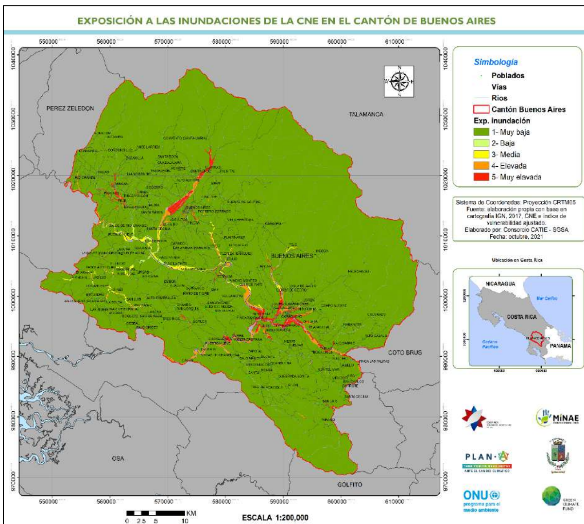
Figura A.5.1. Exposición a las inundaciones de la CNE, en el cantón de Buenos Aires.
