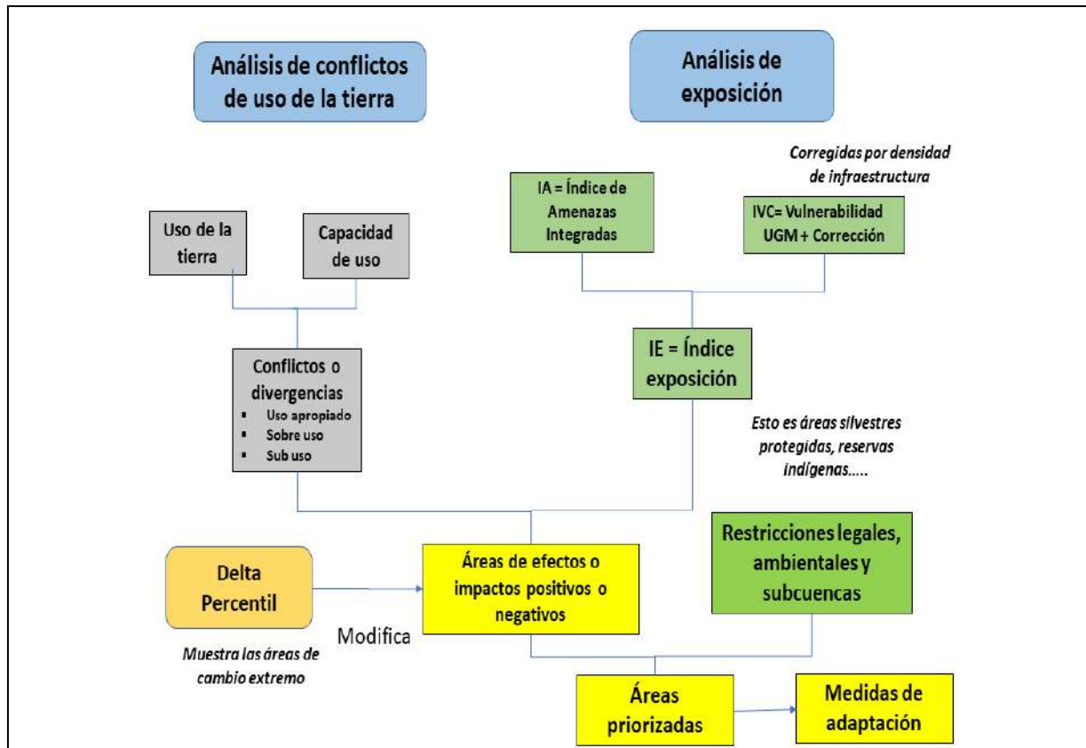
Figura 1. Esquema metodológico propuesto para el desarrollo del análisis de los conflictos en el uso de la tierra y de la exposición ante las amenazas relacionadas con los procesos de origen hidrometeorológico y de la geodinámica externa.
