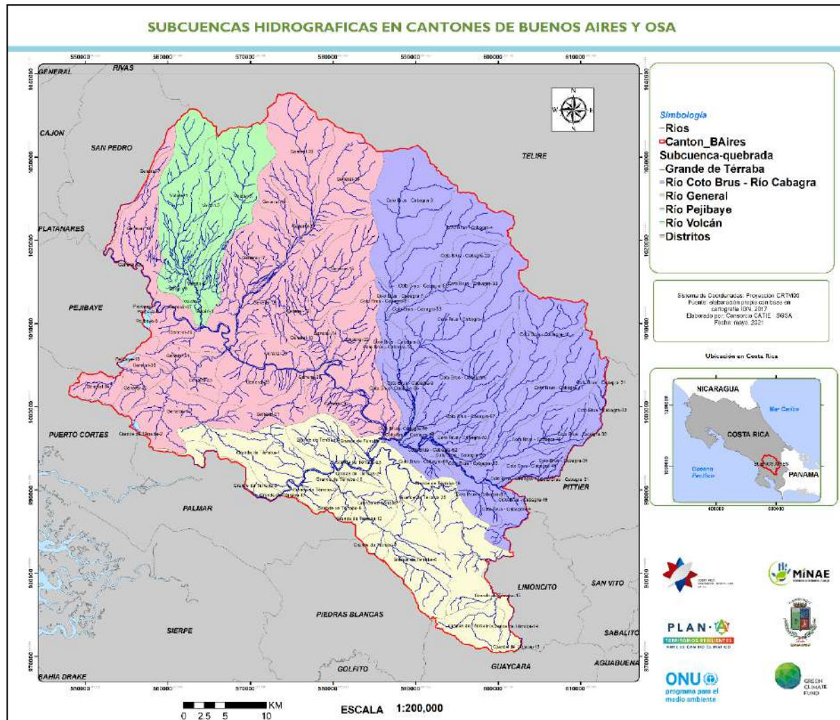
Figura 4. Cantón de Buenos Aires y sistema de drenaje por subcuencas y quebradas Fuente: Elaboración propia con base en SNIT, 2017
