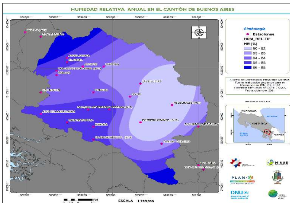
Figura 8. Humedad relativa en el cantón de Buenos Aires Fuente: Elaboración propia, con base en CNE (2013)
