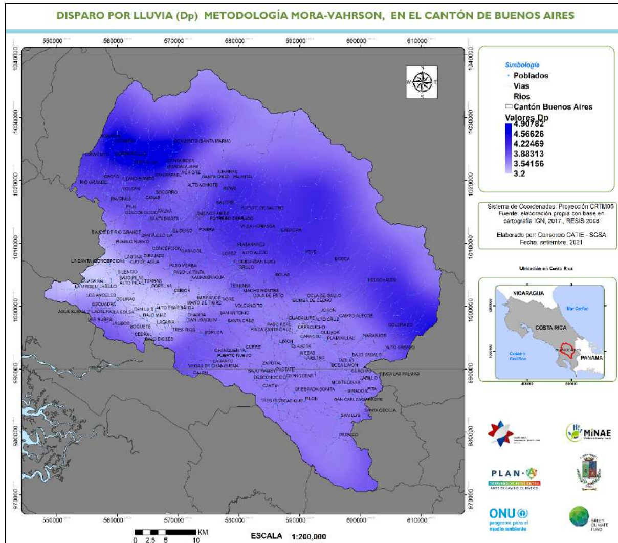
Figura A.2-11. Disparo por intensidad de lluvia (Dp), método Mora & Vahrson, en el cantón de Buenos Aires
