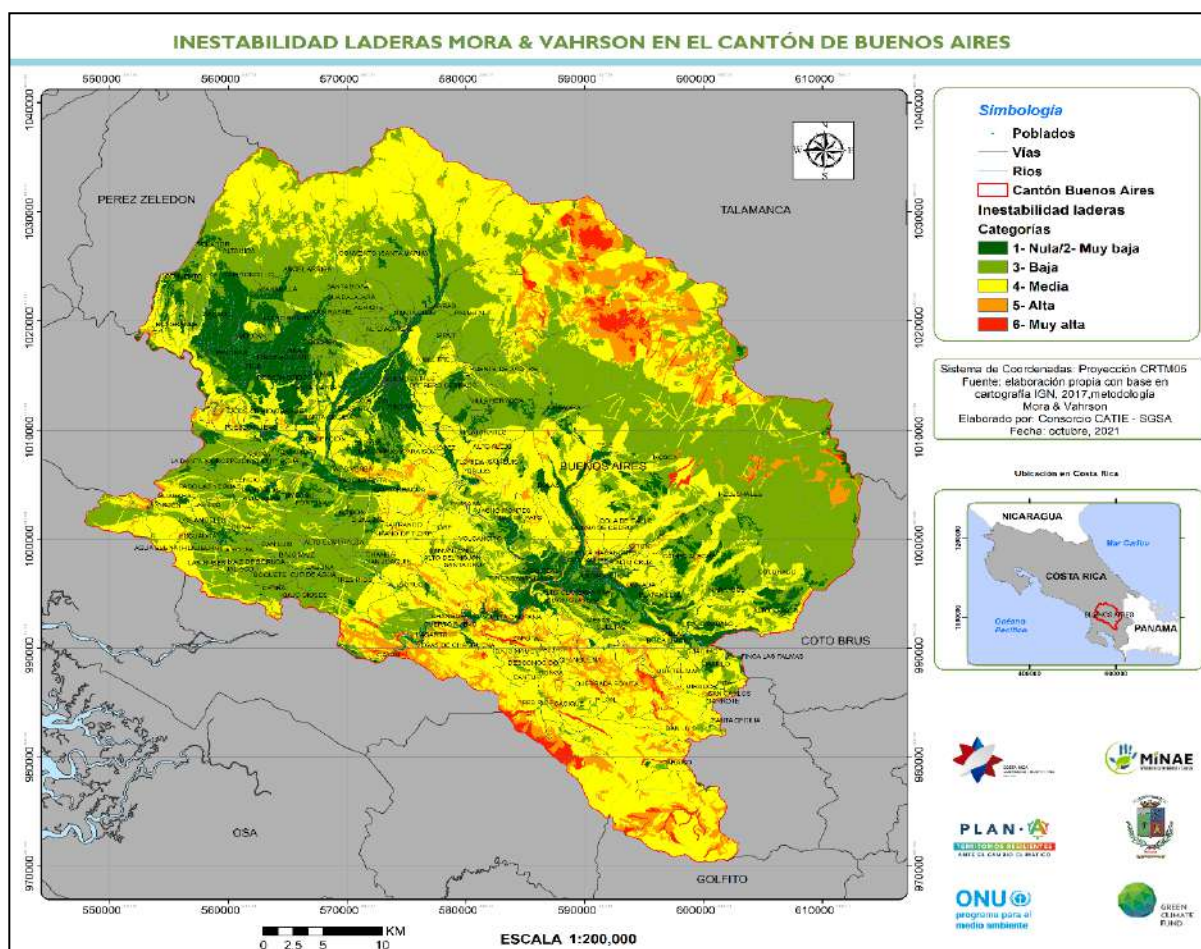
Figura 21. Inestabilidad de laderas en el Cantón de Buenos Aires, a partir de la metodología de Mora y Vahrson (1994)
