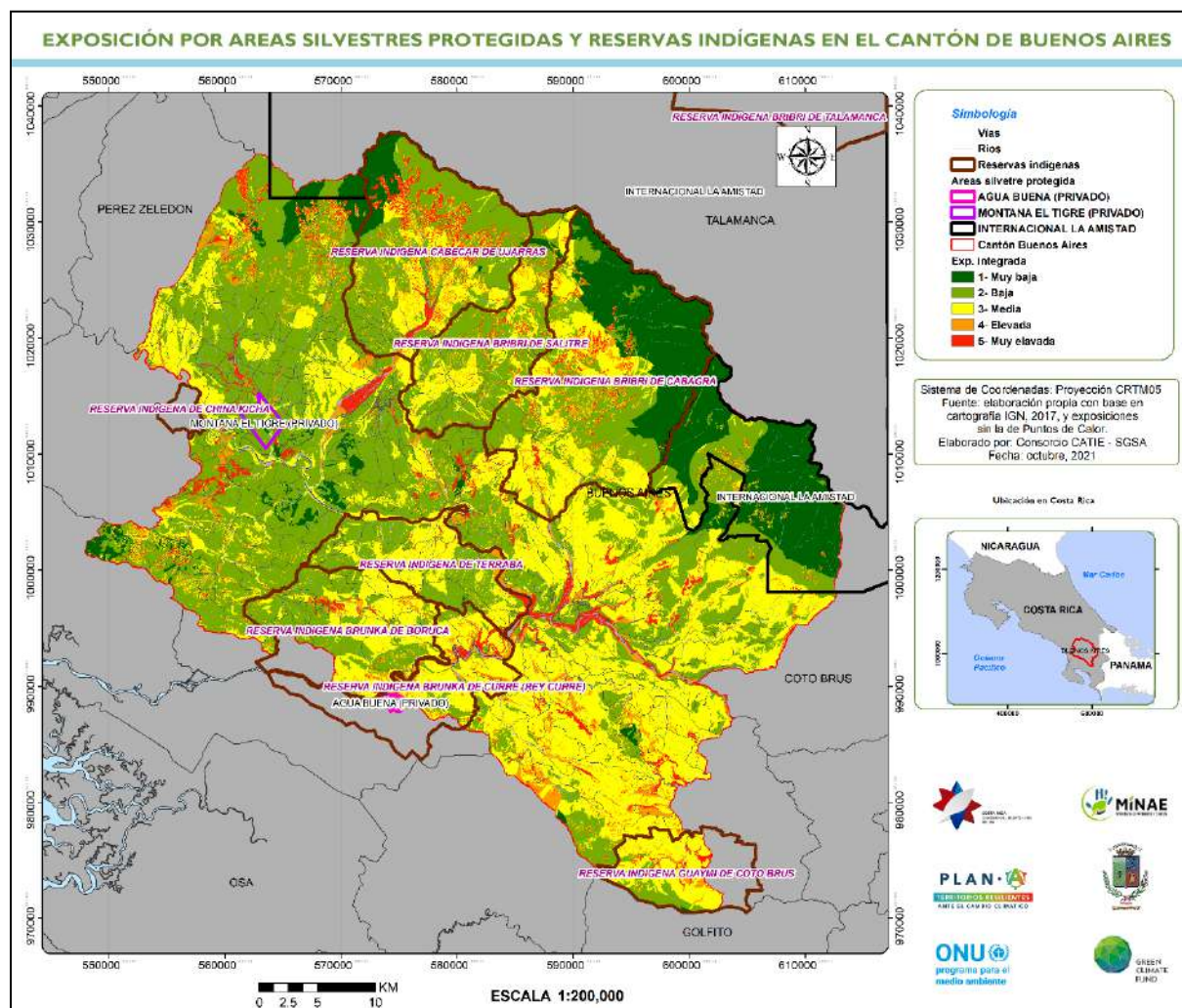
Figura 40. Áreas Silvestres Protegidas y reservas indígenas sobrepuestas a la exposición integrada en el cantón de Buenos Aires
