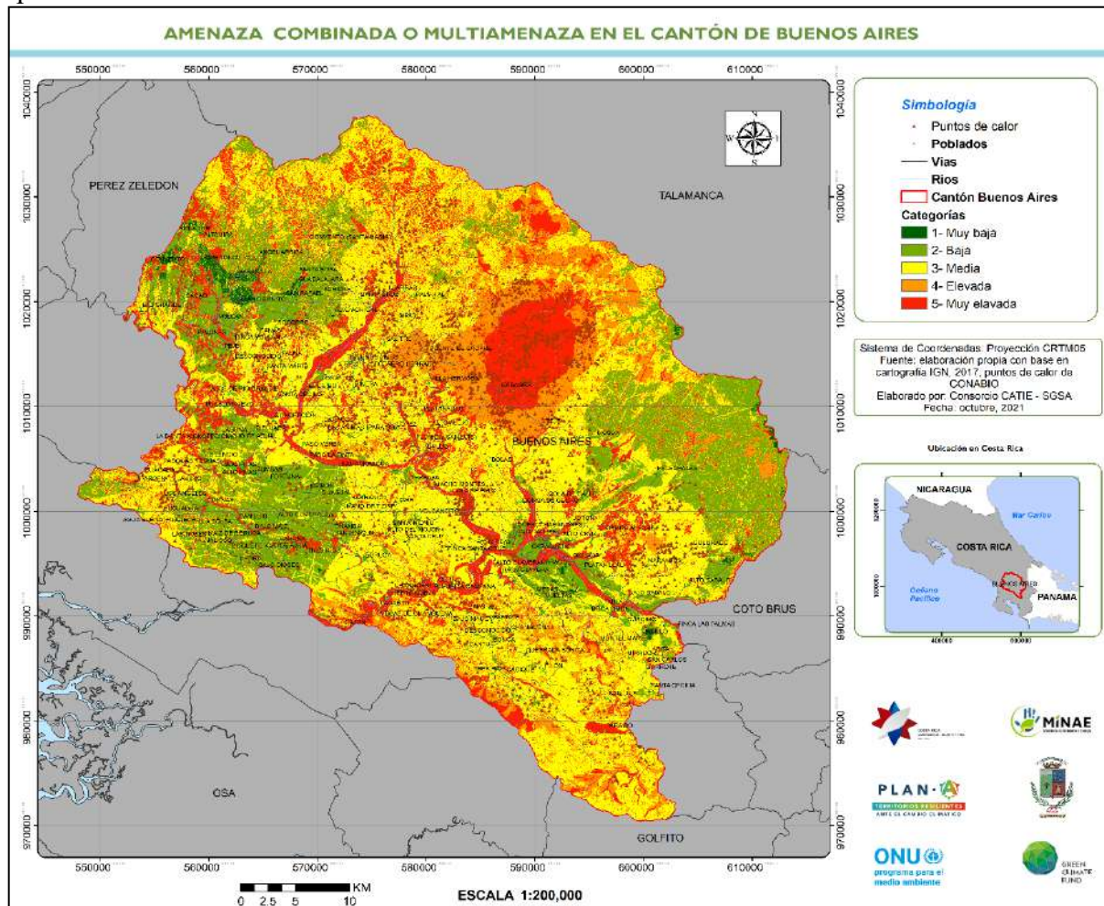
Figura 26. Multiamenazas 13 en el cantón de Buenos Aires
