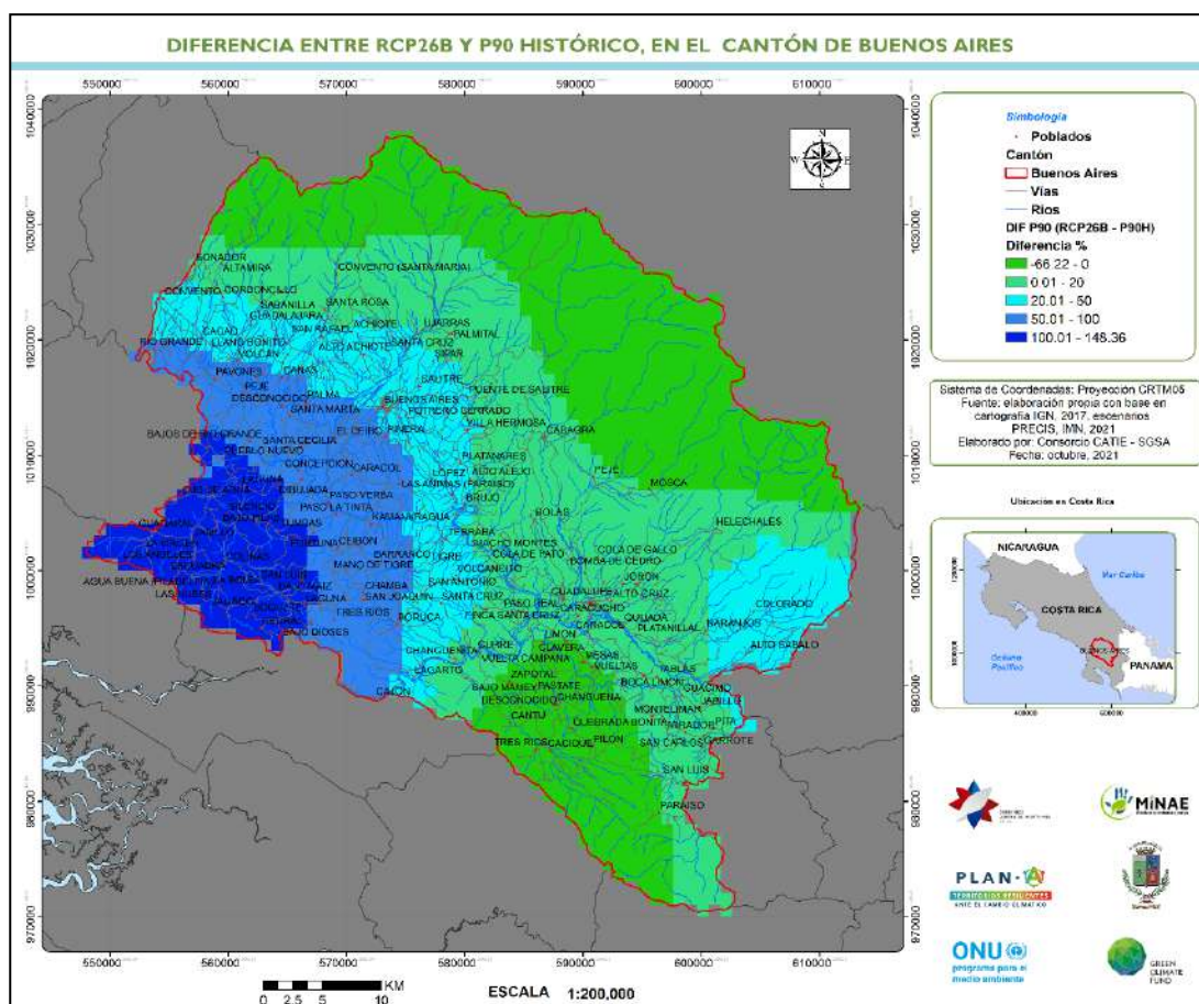
Figura 32. Diferencia del P90_RCP26B respecto P90_Hist, en porcentaje
