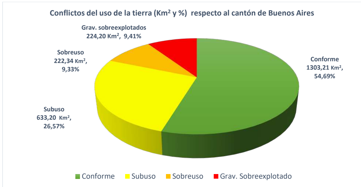
Figura 25. Conflictos del uso de la tierra en el cantón de Buenos Aires
