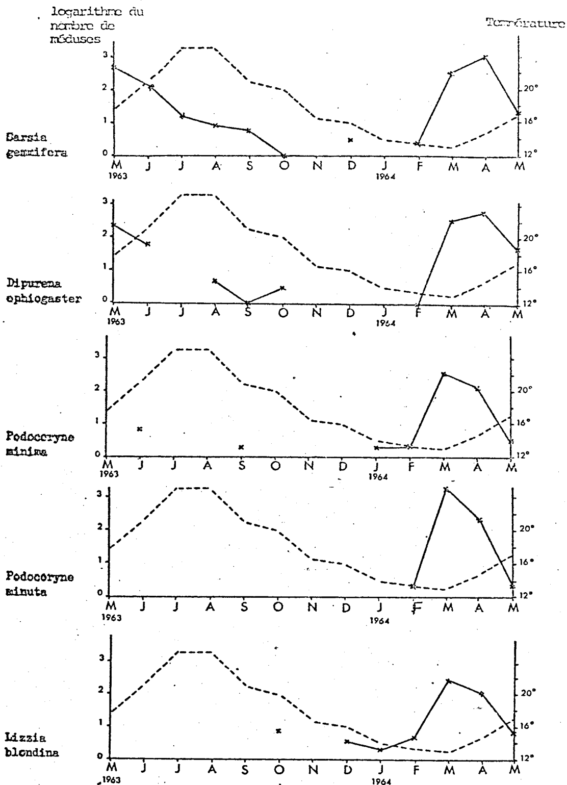
Figure I. Variations, en valeurs logarithmiques, du nombre d'Anthoméduses dans la rade. 1: Sarsia gemmifera ; 2: Dipurena ophiogaster ; 3: Podocoryne minima ; 4: P. minuta ; 5: Lizzia blondina . En pointillé: courbe de temp. moyenne au point B. à 0m.
