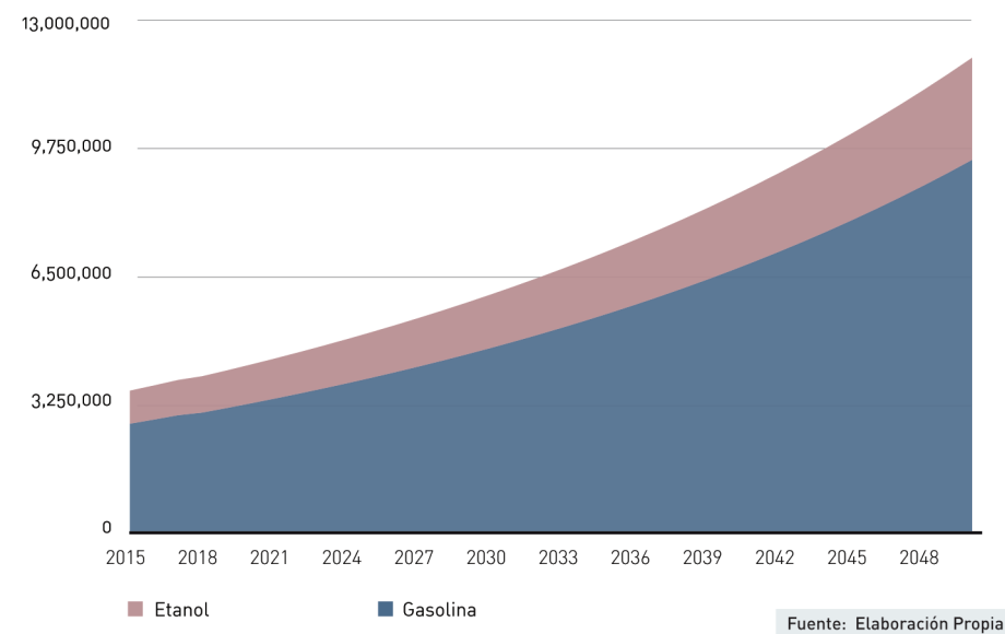
FIGURA 26 Demanda de energía de la flota de vehículos livianos Latinoamérica - Escenario BAU (Unidad: Tjoule)
