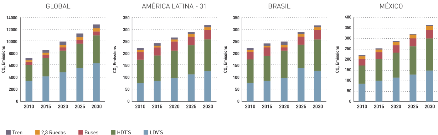
FIGURA 15 Emisiones del sector transporte por región y tipo de vehículo
