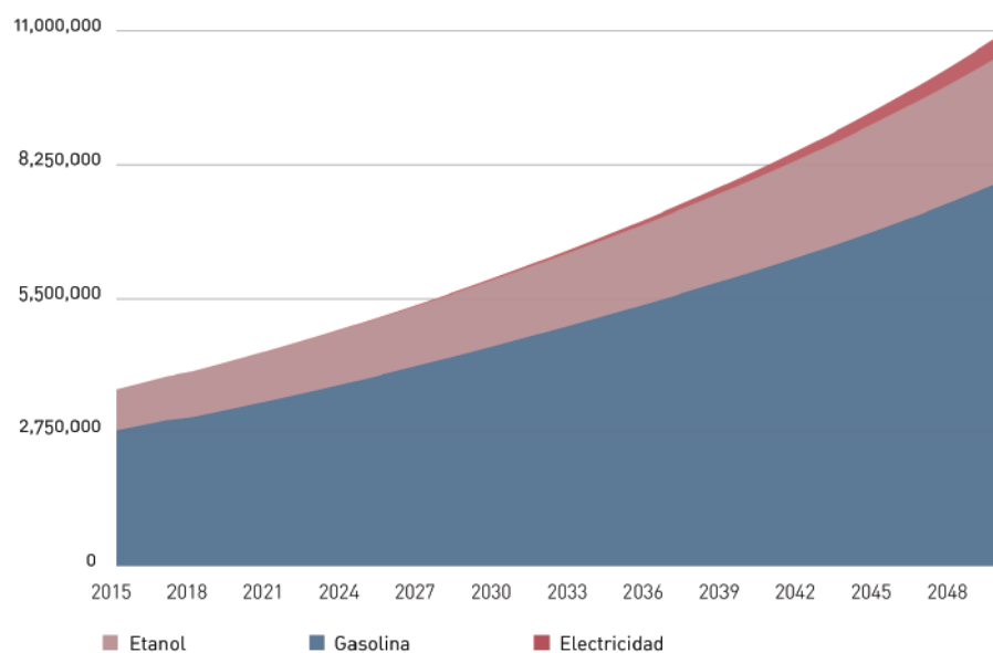
FIGURA 27 Demanda de energía de la flota de vehículos livianos Latinoamérica - Escenario promoción VEs (Unidad: Tjoule)
