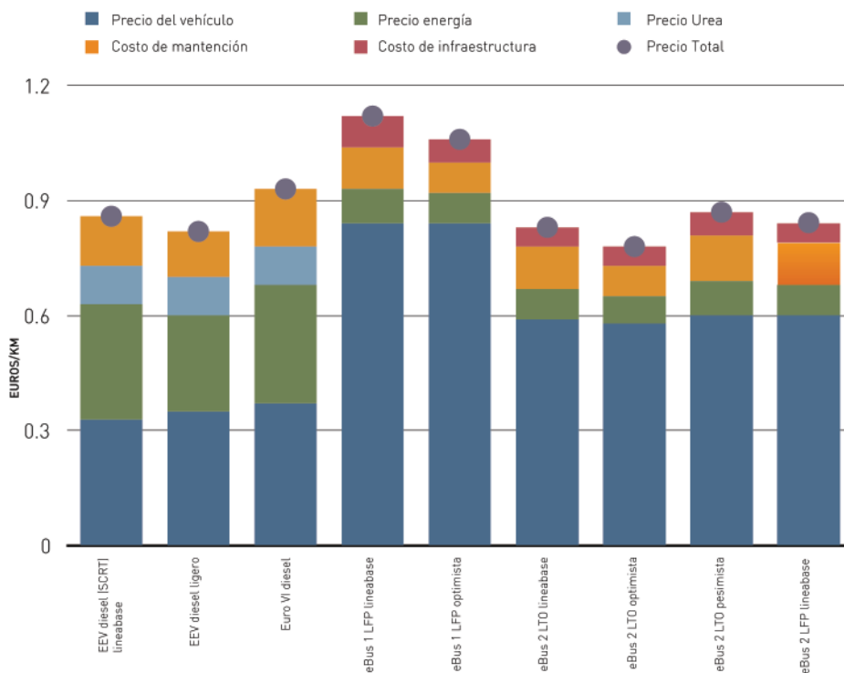
FIGURA 7 Costos totales por kilómetro recorrido y por tipo de bus operando en Finlandia
