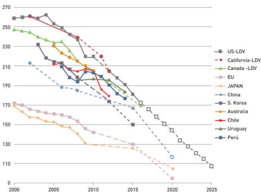
FIGURA 32 Emisiones de CO 2 en la flota de vehículos livianos en distintos países
