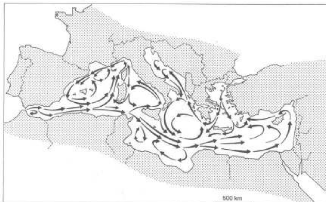
Figure 68 Tendances générales des courants marins de surface en été
