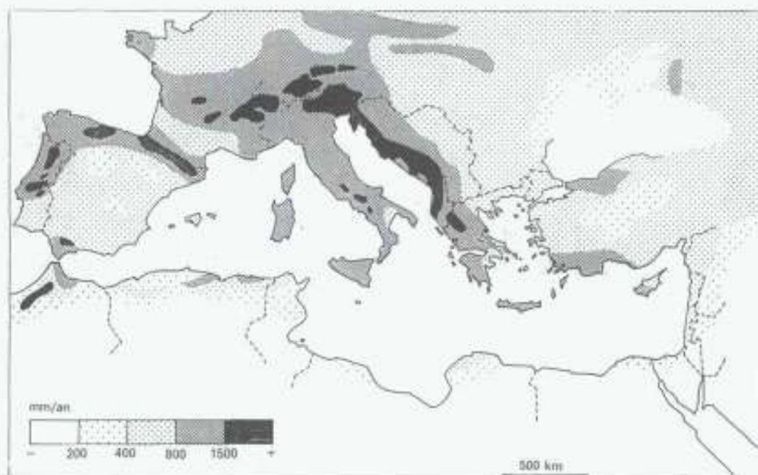
Figure 5 Précipitations moyennes annuelles
