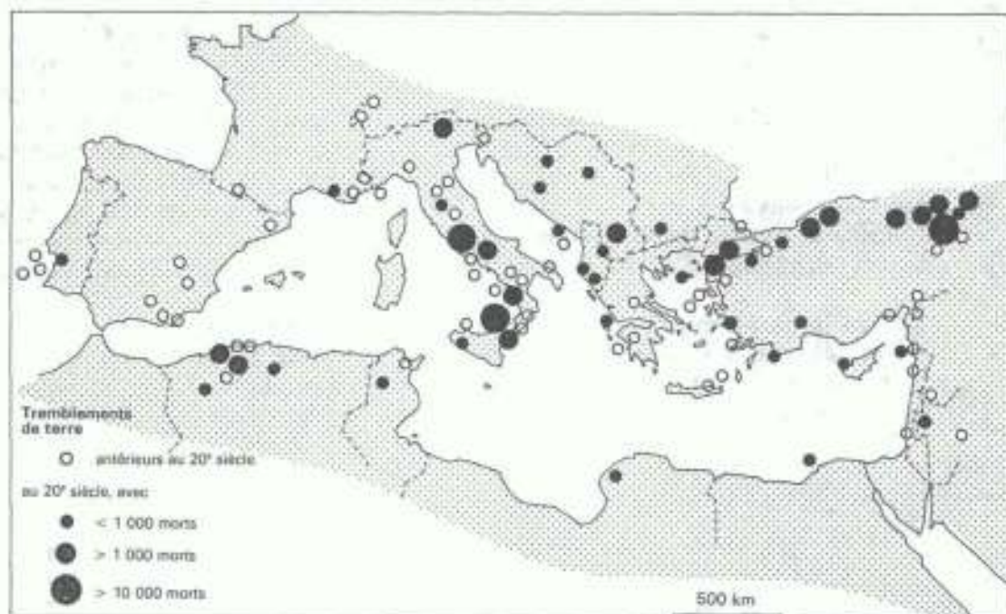
Figure 2 Les tremblements de terre catastrophiques
