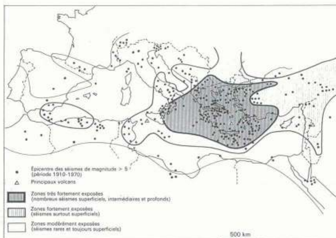
Figure 1 Sismicité et volcanisme
